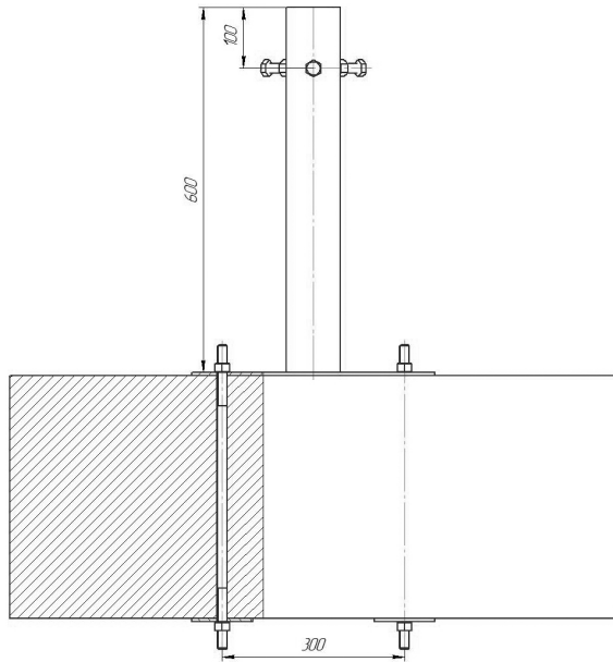
Рисунок 1. Общий вид гильзы ОГР-1
